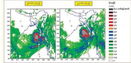
မိုးလေဝသနှင့် ဇလဗေဒညွှန်ကြားမှုဦးစီးဌာန WRF မော်ဒယ်လ်၏ ၂၀-၁၀-၂၀၂၄ ရက်နေ့ မြန်မာစံတော်ချိန် (၀၆:၃၀) နာရီအချိန်ကို အခြေခံတွက်ထုတ်ထားသည့် ၂၁-၁၀-၂၀၂၄ မှ ၂၂-၁၀-၂၀၂၄ ရက်နေ့အထိ မိုးရွာသွန်းမှုခန့်မှန်းချက်ပြပုံ
